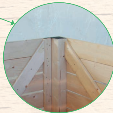
detail vnútra - rohový hranol
