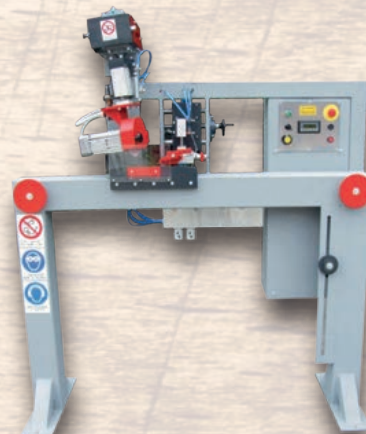
automatische Schleifmaschine
