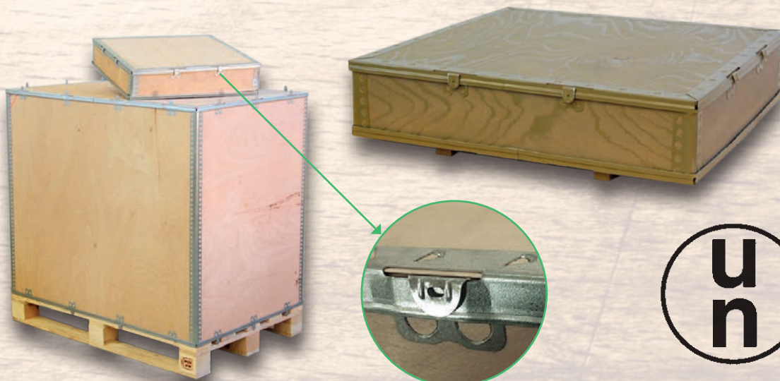
Detail Zungenschlitze und Stahlzunge
